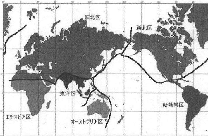
図2 動物の分布を制限する地理的障壁によって区分された動物地理区
