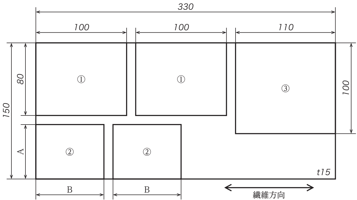
材料取り図
